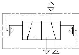
ANSI Symbol
